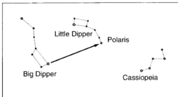
Fig. 7: Locating Polaris.
